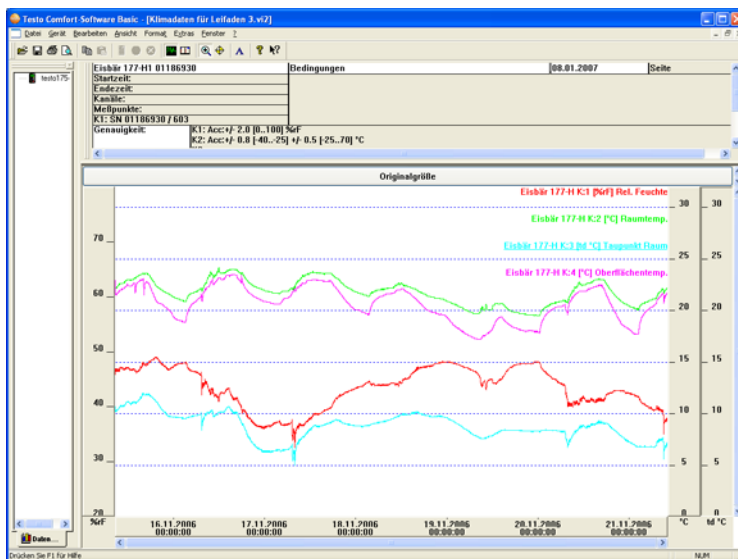
Abb.2 Aufzeichnung Raumklima: Temperatur, Feuchte und Taupunkt der Luft
