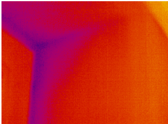
Abb.1 Thermografische Aufnahme einer Außenwanddecke (dunkel = kalt)
